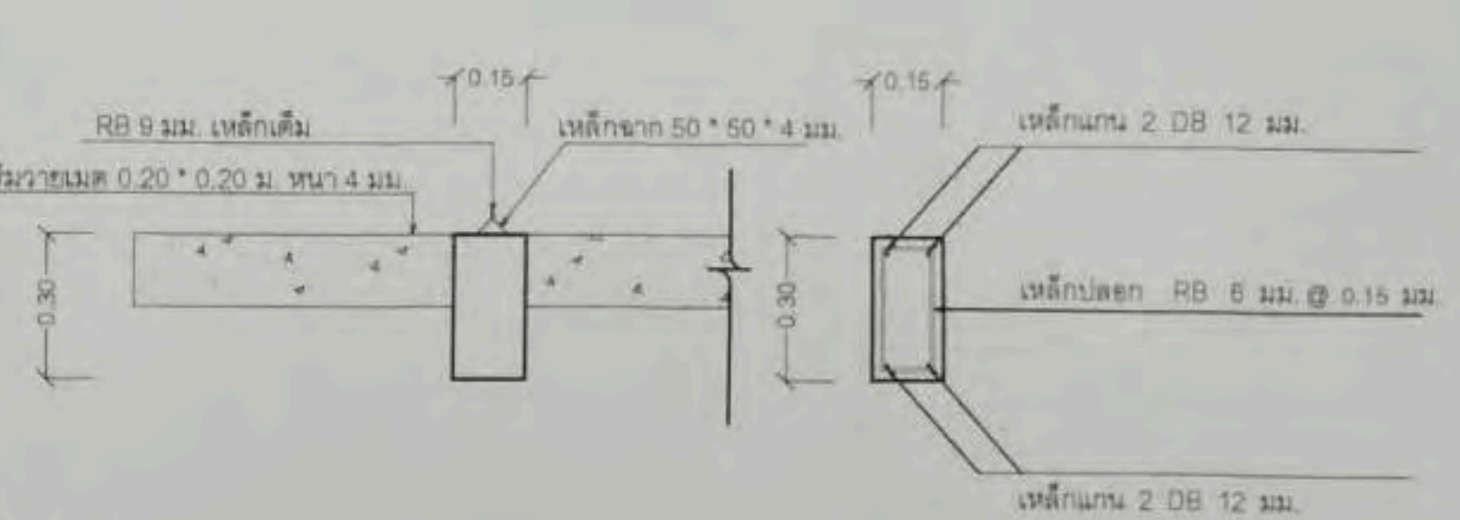
รูปตัดขยาย คานคอดินรับประตู NO SCALE
